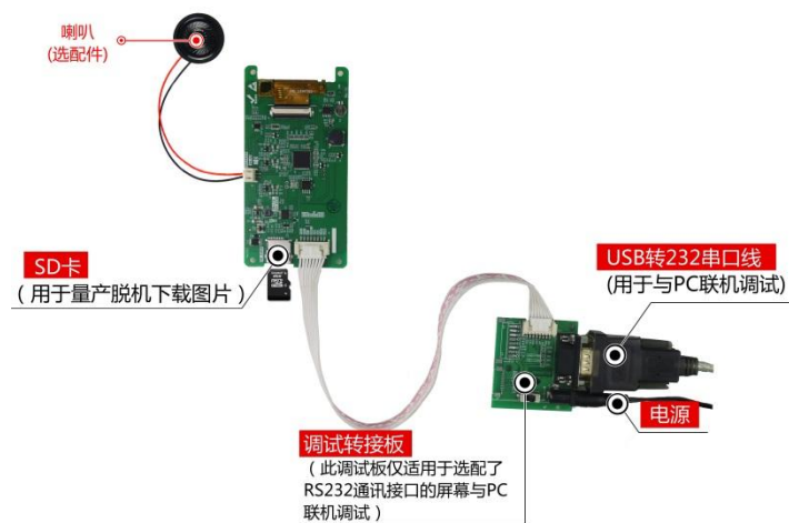
图 1-3 调试工具图
