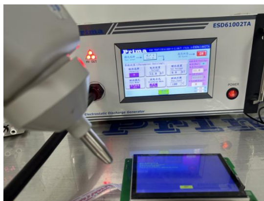
图 5-2 ESD 测试图
